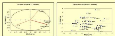
Figure 6: Analyse en composantes principales de la diversité de Shannon, du cumul de CO 2 , de l'azote minéral et du ratio C/N
