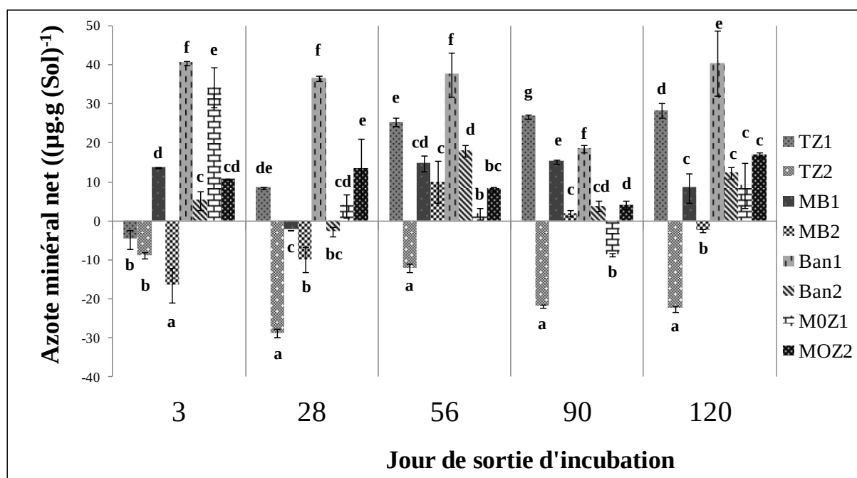
Figure 8 : Minéralisation nette de l'azote des sols amendés avec les feuilles de Jatropha des différentes provenances (TZ=Tanzanie ; MOZ=Mozambique ; Ban=Banfadjiré ; MB=Madiop Boye ; 1 =feuilles vertes ; 2 =feuilles jaunes ; pour chaque sortie d'incubation, les lettres différentes indiquent des valeurs significativement différentes : p < 0,05 ).
