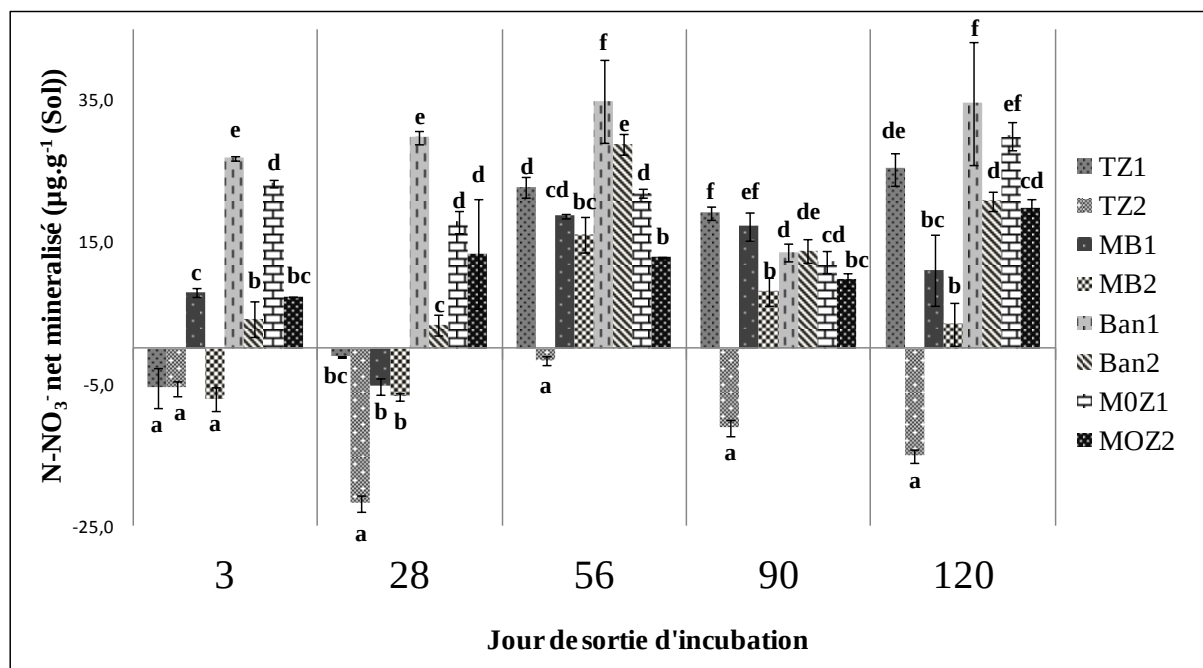
Figure 9 : Nitrification des sols amendés avec les feuilles de Jatropha des différentes provenances (TZ=Tanzanie ; MOZ=Mozambique; Ban=Banfadjiré; MB=Madiop Boye ; 1=feuilles vertes ; 2=feuilles jaunes ; pour chaque sortie d'incubation, les lettres différentes indiquent des valeurs significativement différentes : p < 0,05 ).
