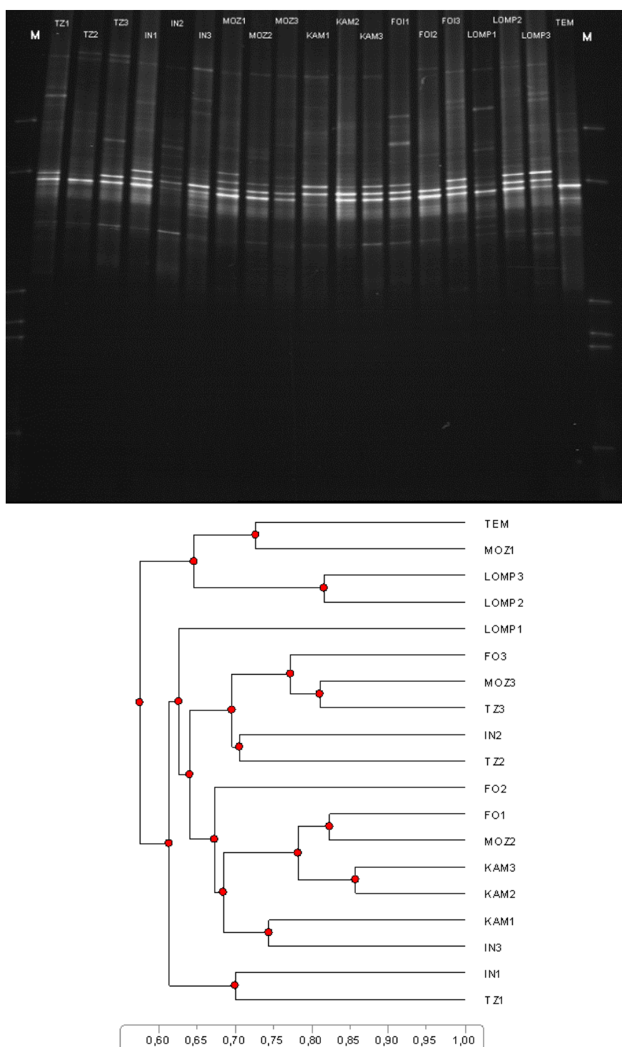
Figure 16 : Gel DGGE (haut) et dendrogramme de similarité (bas) des communautés bactériennes nitrifiantes de la rhizosphère de Jatropha des différentes provenances (IN: Inde, TZ: Tanzanie, MOZ: Mozambique, FO : Fois 1, KAM : Kamonghone, LOMP : Lompoul, TEM : Témoin).
