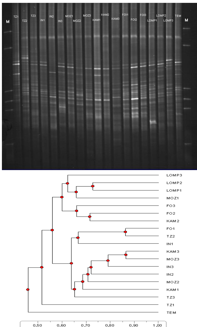
Figure 17 : Gel DGGE (haut) et dendrogramme de similarité (bas) des communautés bactériennes dénitrifiantes de la rhizosphère de Jatropha des différents provenances (IN: Inde, TZ: Tanzanie, MOZ: Mozambique, FO : Fois 1, KAM: Kamonghone, LOMP : Lompoul, TEM : Témoin).
