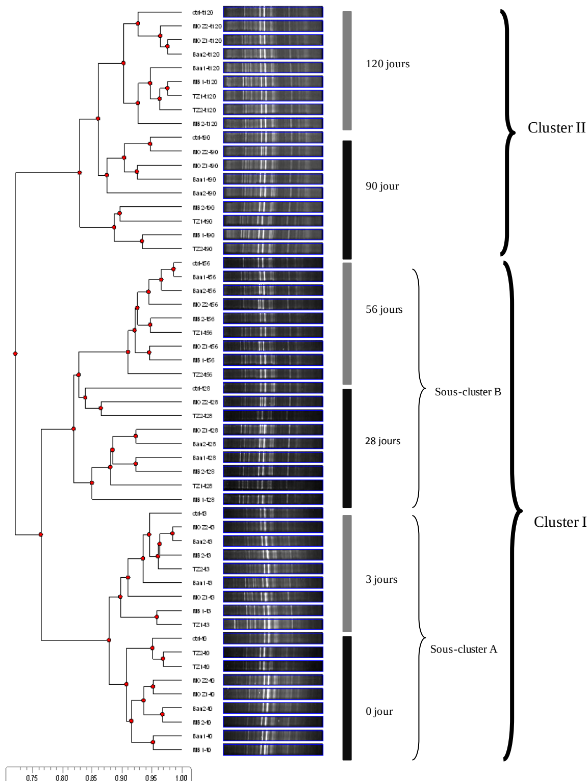
Figure 11 : Dendrogramme UPGMA des communautés bactériennes à 0, 3, 28, 56, 90 et 120 jours (Ban=Banfadjiré ; MB= Madiop Boye ; MOZ=Mozambique ; Ctrl=témoin ; TZ=Tanzanie ; 1=résidu vert et 2=résidu jaune).
