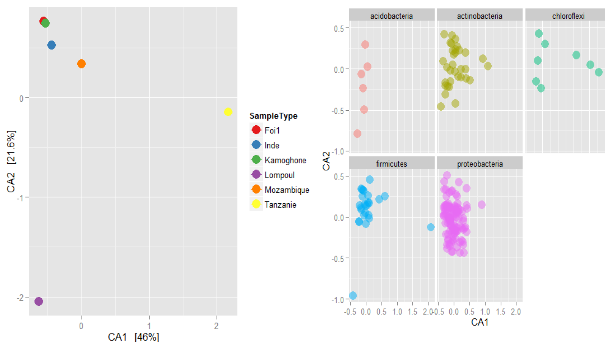
Figure 42 : Analyse en correspondance pour les 5 phyla les plus abondants des 200 OTU les plus abondantes de la rhizosphère des différentes provenances de Jatropha .
