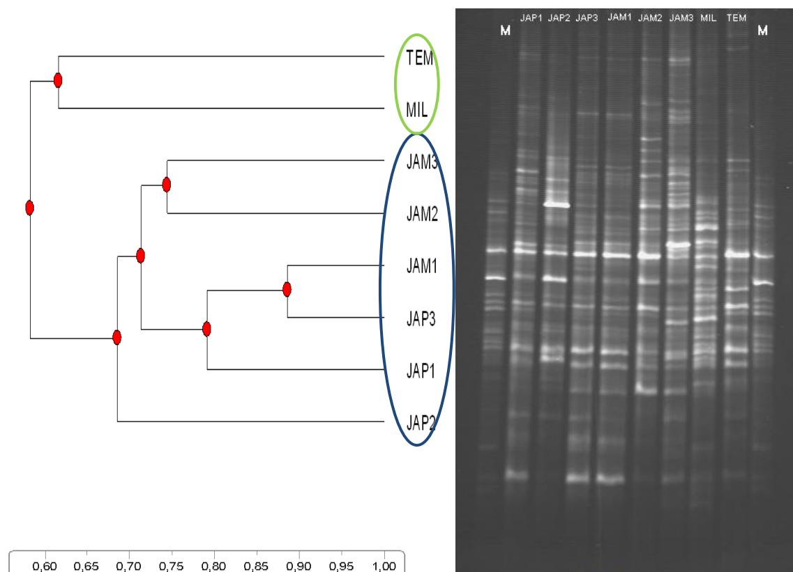
Figure 27 : Gel DGGE (droite) et dendrogramme de similarité (gauche) des communautés fongiques de la rhizosphère de Jatropha des différents systèmes de culture (JAP=culture pure de Jatropha , JAM= Jatropha en association avec le mil), celle du mil (MIL) et du témoin non cultivé (TEM).
