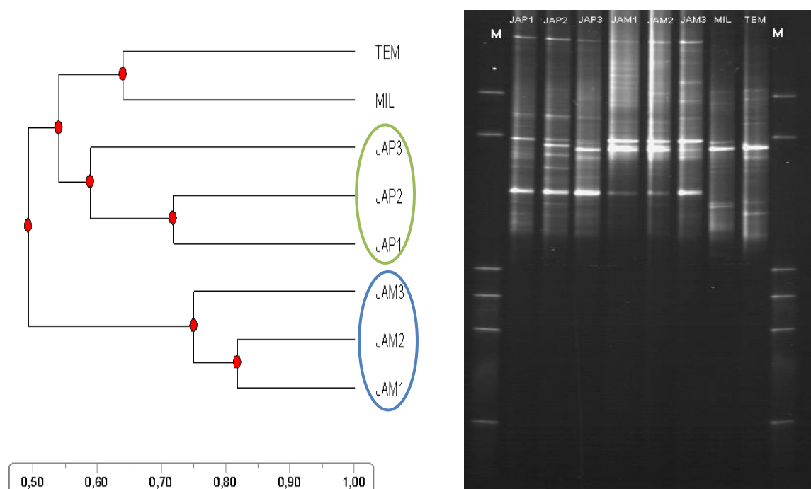
Figure 20 : Gel DGGE (droite) et dendrogramme de similarité (gauche) des communautés nitrifiantes de la rhizosphère de Jatropha des différents systèmes de culture (JAP=culture pure de Jatropha , JAM= Jatropha en association avec le mil), celle du mil (MIL) et du témoin non cultivé (TEM).
