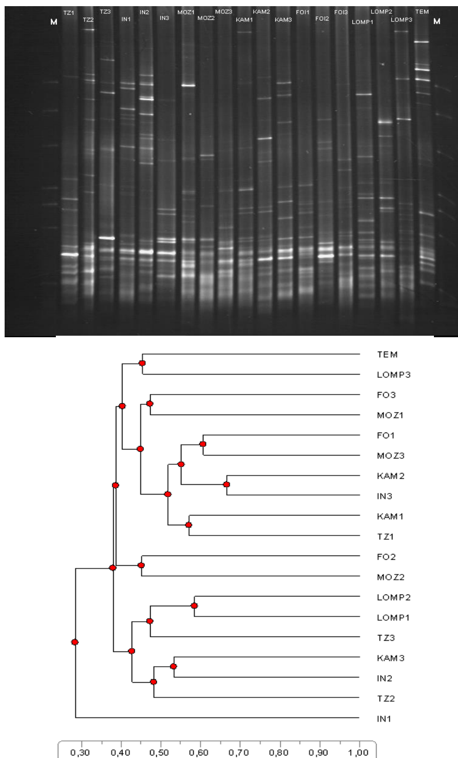
Figure 18 : Gel DGGE (haut) et dendrogramme de similarité (bas) des communautés bactériennes fixatrices d'azote de la rhizosphère de Jatropha des différentes provenances (IN: Inde, TZ : Tanzanie, MOZ : Mozambique, FO : Fois 1, KAM : Kamonghone, LOMP : Lompoul, TEM : Témoin).
