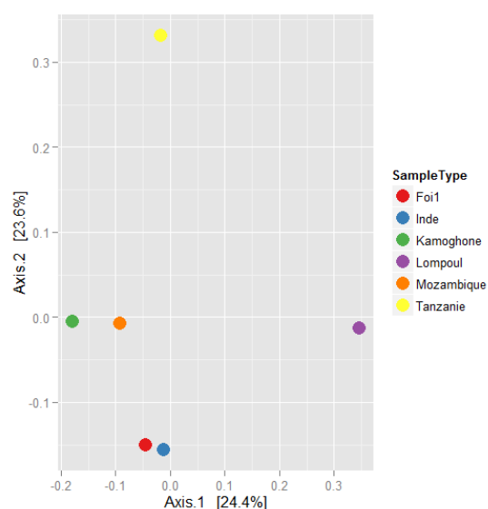
Figure 39 : MDS pour les Acidobactéria de la rhizosphère de Jatropha des provenances Foi 1, Kamonghone, Lompoul, Inde, Mozambique et Tanzanie.
