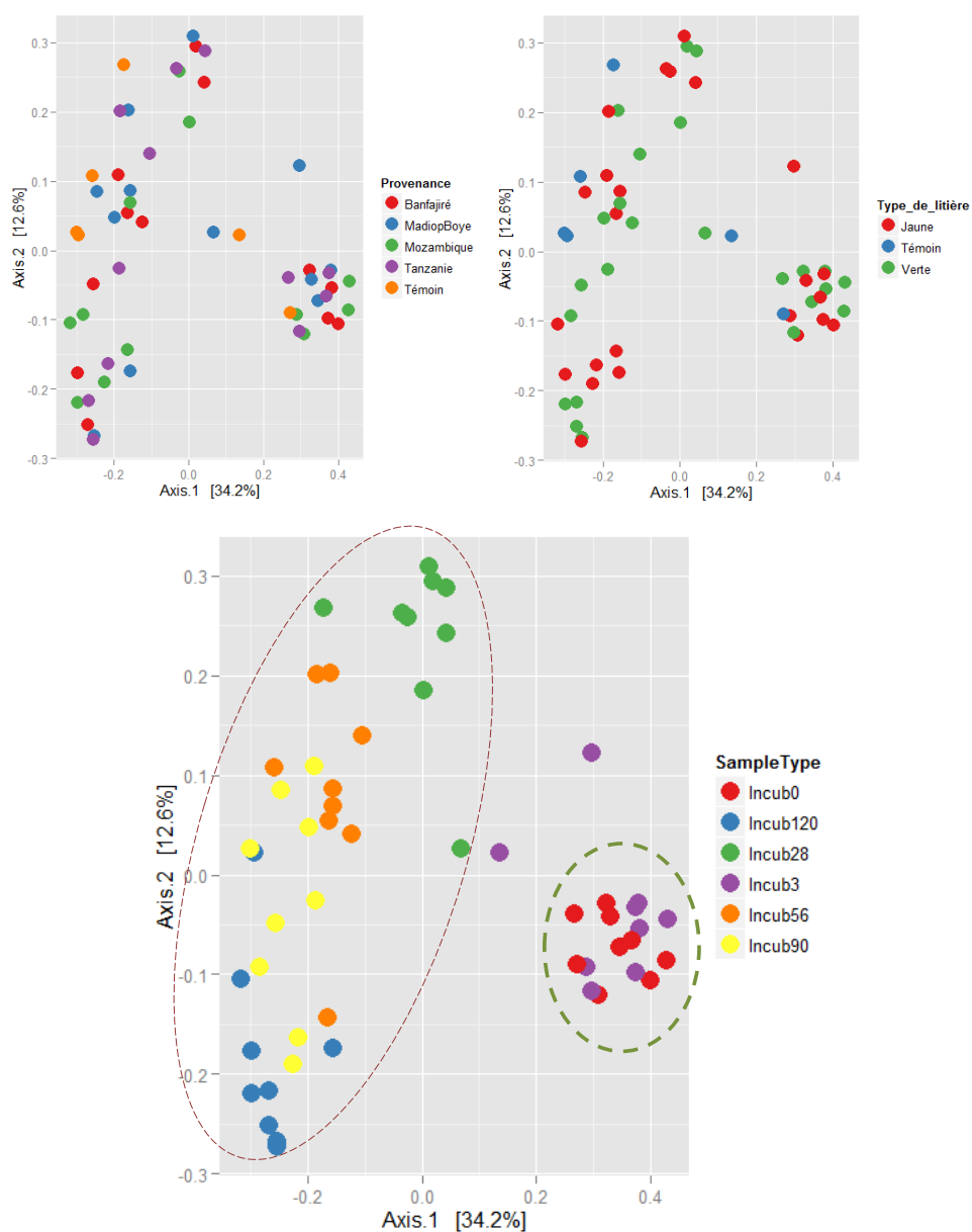
Figure 33: MDS pour le phylum Protéobactéria en fonction des provenances de Jatropha , du degré de maturité des feuilles (type de litière) et du temps d'incubation (Sample Type).
