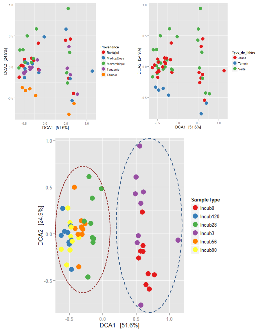
Figure 30: DCA des sols en fonction de la durée de l'incubation, du type de litière et de la provenance.
