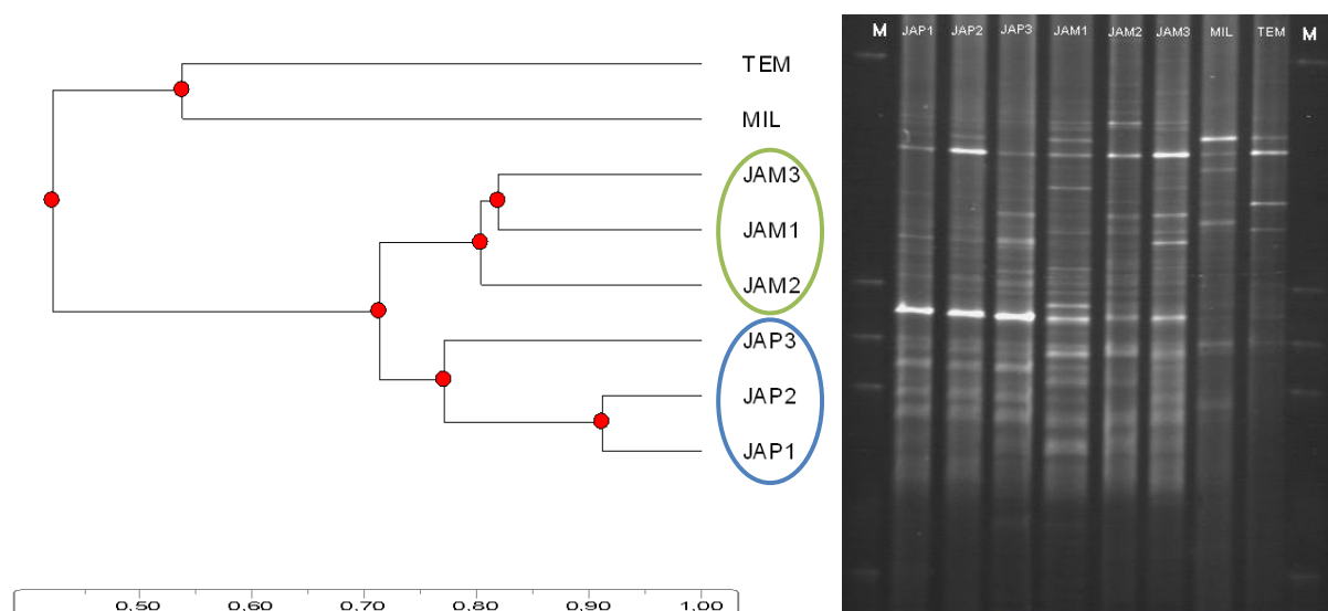
Figure 23 : Gel DGGE (droite) et dendrogramme de similarité (gauche) des communautés dénitrifiantes de la rhizosphère de Jatropha des différents systèmes de culture (JAP=culture pure de Jatropha , JAM= Jatropha en association avec le mil), celle du mil (MIL) et du témoin non cultivé (TEM).
