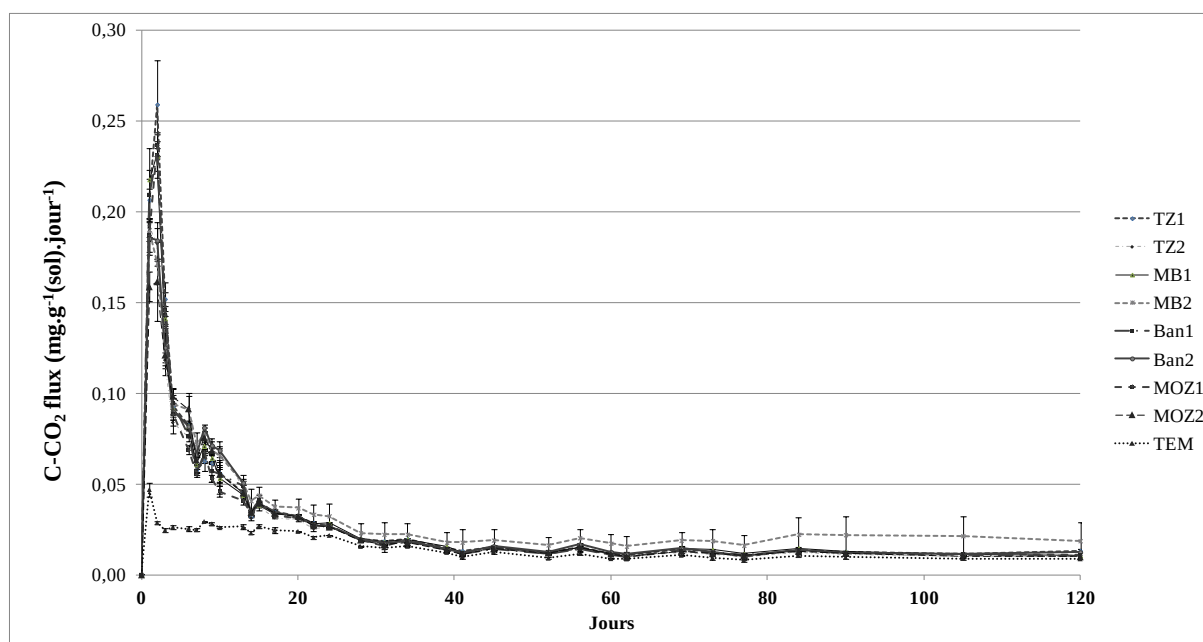
Figure 3 : Flux de CO 2 en mg.g (sol) -1 .jour -1 des sols amendés avec les feuilles de Jatropha des provenances Tanzanie (TZ1 : vert ; TZ2 : jaune), Mozambique (MOZ1 : vert ; MOZ2 : jaune), Banfadjiré (Ban1 : vert ; Ban2 : jaune) et Madiop Boye (MB1 : vert ; MB2 : jaune) et des sols non amendés (TEM : Témoin).
