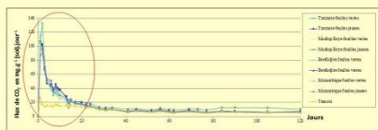
Figure 5: Activité respiratoire mesurée des sols sous l'influence de différents types de litières de Jatropha curcas
