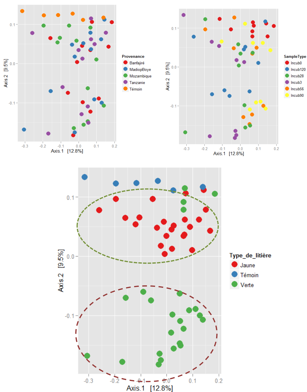
Figure 31: MDS pour le Phylum des Firmicutes en fonction des provenances de Jatropha , du degré de maturité des feuilles (type de litière) et du temps d'incubation (Sample Type).
