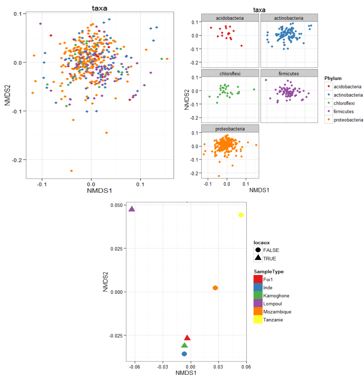
Figure 41 : NMDS des rhizosphères des différentes provenances de Jatropha et des 5 phyla les plus abondants (Acidobactéria, Actinobactéria, Chloroflexi, Firmicutes et Protéobactéria).
