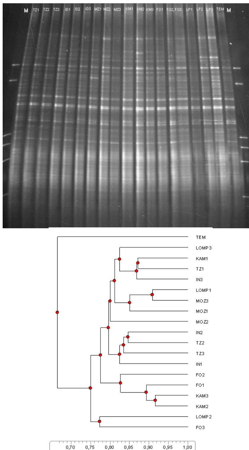
Figure 14 : Gel DGGE (haut) et dendrogramme de similarité (bas) des communautés bactériennes de la rhizosphère de Jatropha des différentes provenances (IN : Inde, TZ : Tanzanie, MOZ : Mozambique, FO : Fois 1, KAM : Kamonghone, LOMP : Lompoul, TEM : Témoin).
