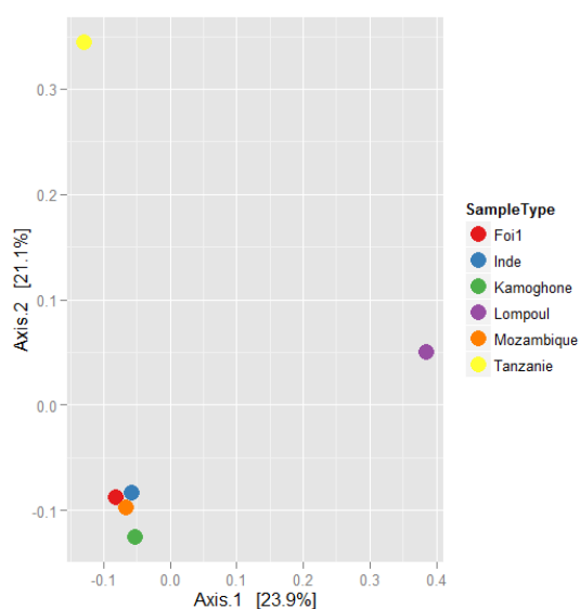
Figure 37 : MDS pour les Firmicutes de la rhizosphère de Jatropha des provenances Foi 1, Kamonghone, Lompoul, Inde, Mozambique et Tanzanie.
