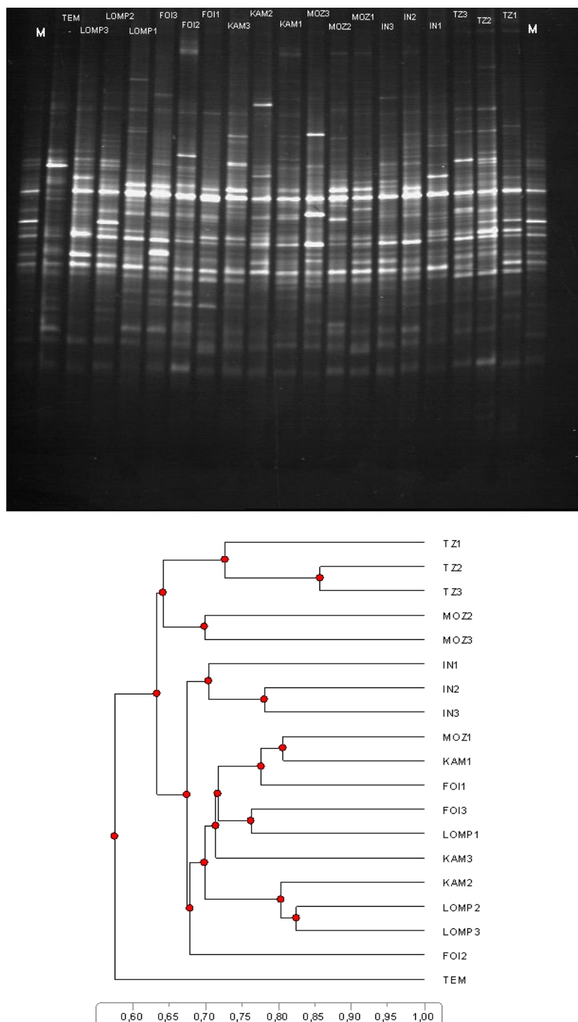
Figure 15 : Gel DGGE (haut) et dendrogramme de similarité (bas) des communautés fongiques de la rhizosphère de Jatropha des différentes provenances (IN : Inde, TZ : Tanzanie, MOZ : Mozambique, FO : Fois 1, KAM: Kamonghone, LOMP : Lompoul, TEM : Témoin).
