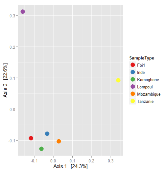
Figure 40 : MDS pour les Actinobactéria de la rhizosphère de Jatropha des provenances Foi 1, Kamonghone, Lompoul, Inde, Mozambique et Tanzanie.
