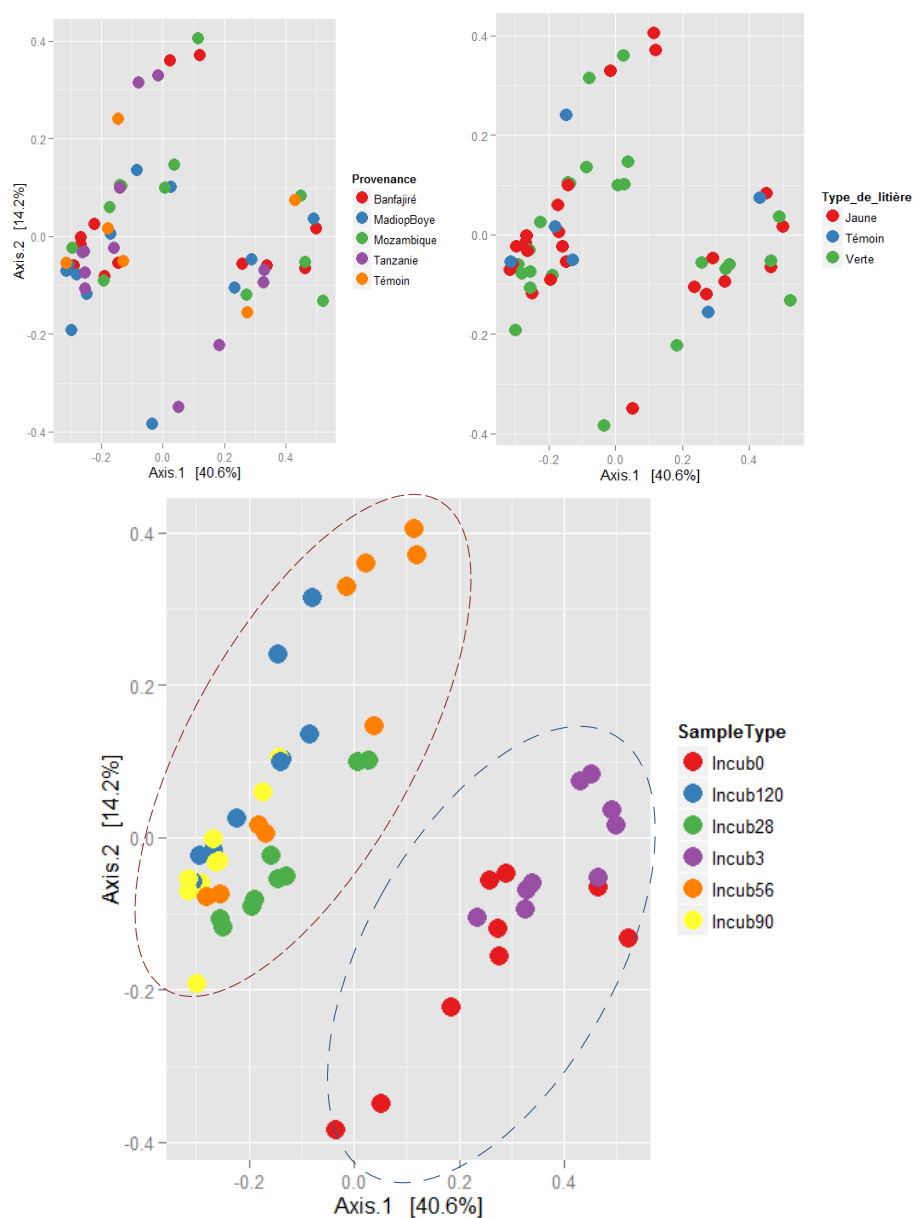
Figure 32: MDS pour le phylum des Acidobacteria en fonction des provenances de Jatropha , du degré de maturité des feuilles (type de litière) et du temps d'incubation (Sample Type).
