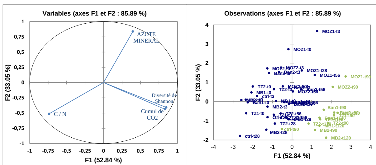
Figure 12: Analyse en composante principale des variables azote minéral, ratio C/N, le cumul des dégagements de CO 2 et la diversité de Shannon des différents traitements au cours du temps.
