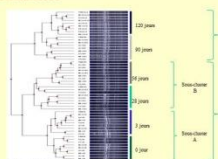
Figure 4: Dendrogramme UPGMA des communautés bactériennes au cours du temps
