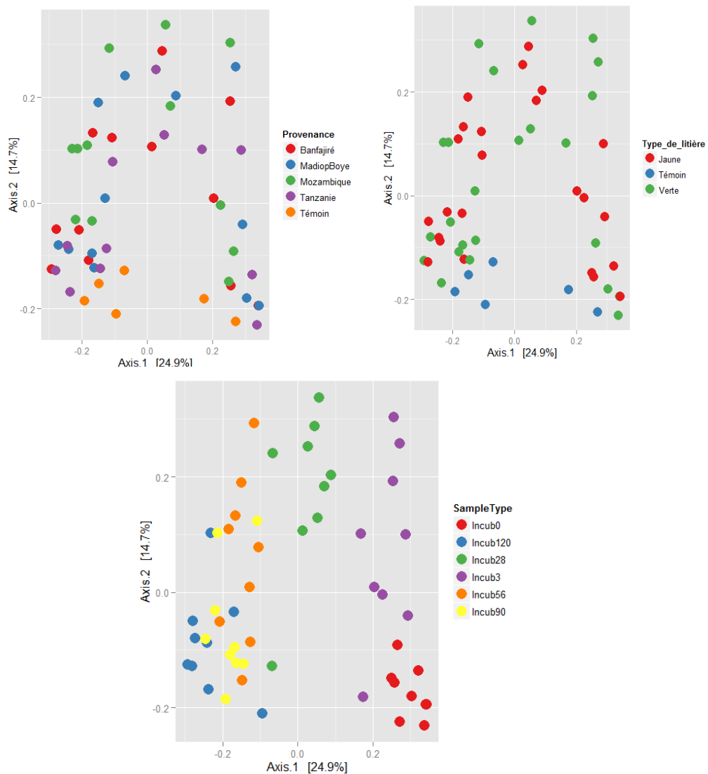
Figure 34 : MDS pour le phylum des Actinobactéria en fonction des provenances de Jatropha , du degré de maturité des feuilles (type de litière) et du temps d'incubation (Sample Type).
