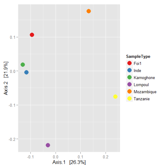
Figure 38 : MDS pour les Protéobactéria de la rhizosphère de Jatropha des provenances Foi 1, Kamonghone, Lompoul, Inde, Mozambique et Tanzanie.
