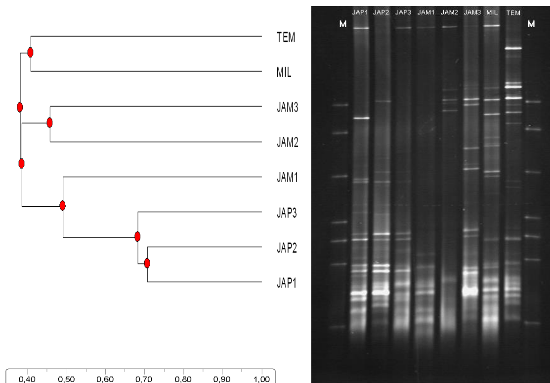
Figure 25 : Gel DGGE (droite) et dendrogramme de similarité (gauche) des communautés fixatrice d'azote de la rhizosphère de Jatropha des différents systèmes de culture (JAP=culture pure de Jatropha , JAM= Jatropha en association avec le mil), celle du mil (MIL) et du témoin non cultivé (TEM).
